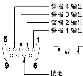
警报连接器
