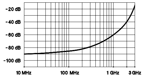
串扰 (75Ω)
