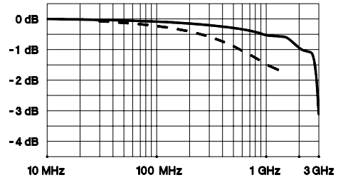
插入损耗 (75Ω)
