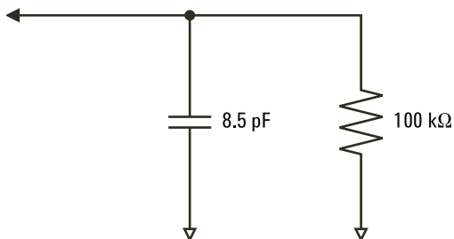
图 23 直流和低频探头等效电路
