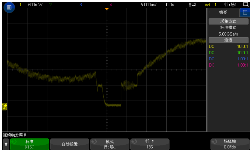
图 29 例如：在行 136 上触发
