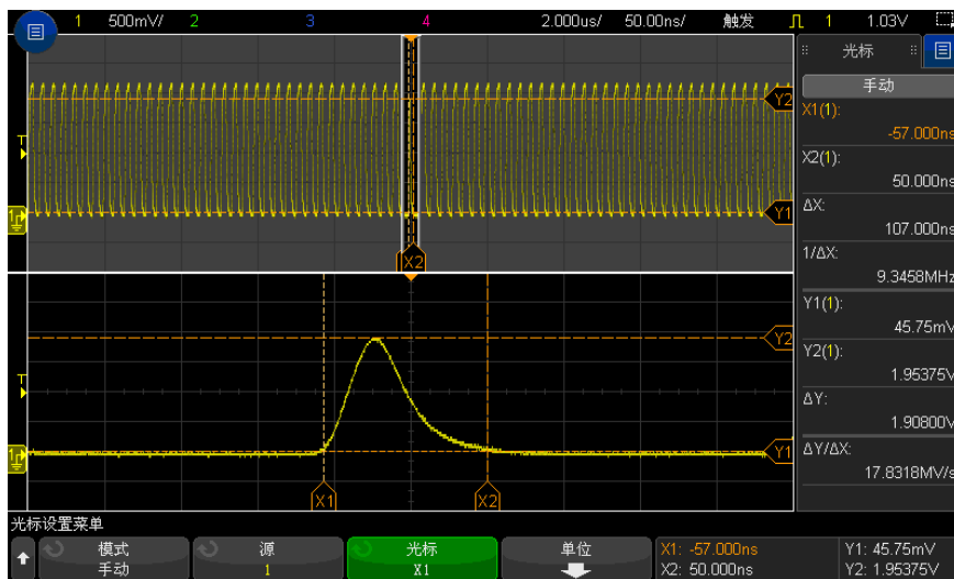
图 44 光标跟踪缩放窗口视图
