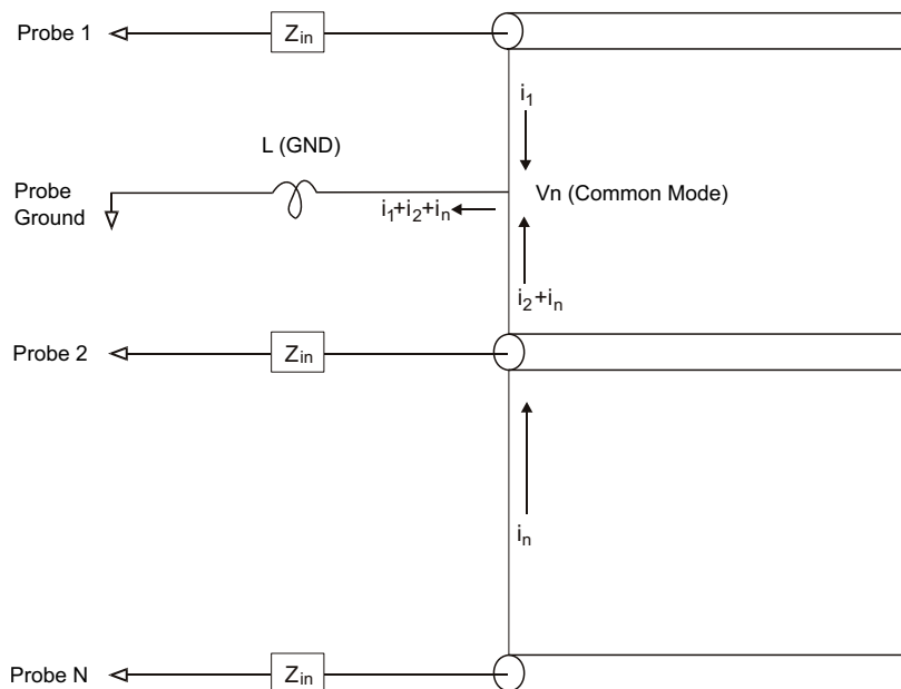
图 26 共模输入电压模型
