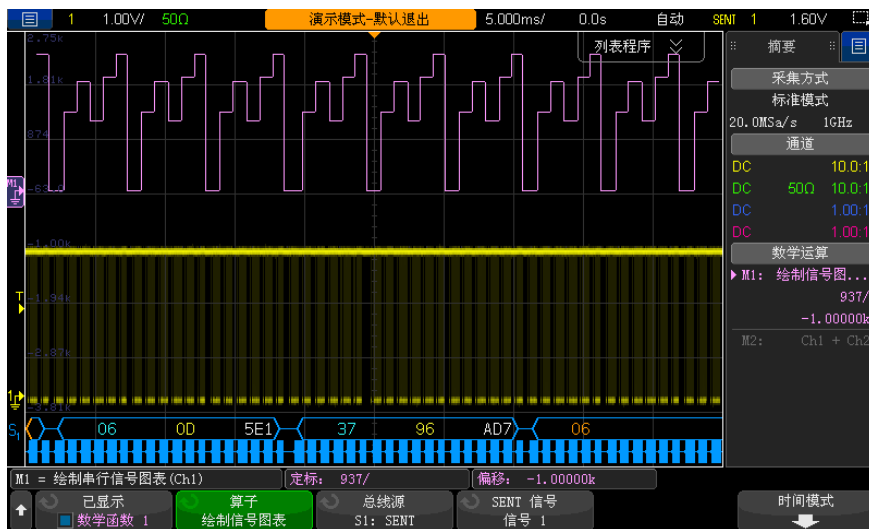
图 21 绘制串行信号图表示例
