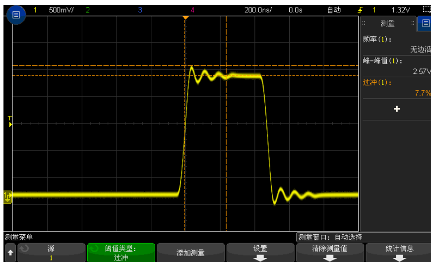
图 49 自动过冲测量
