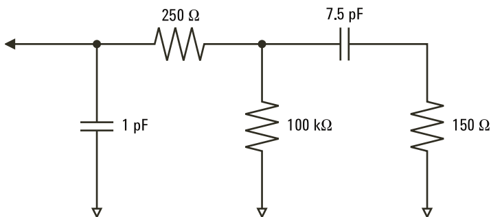
图 24 高频探头等效电路
