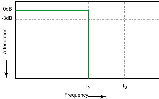
图 36 理论上的砖墙频率响应
