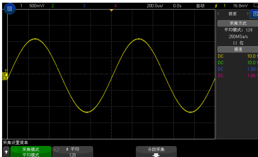
图 41 用于降低随机噪声的平均数 128
