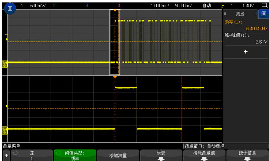
图 50 隔离频率测量事件
