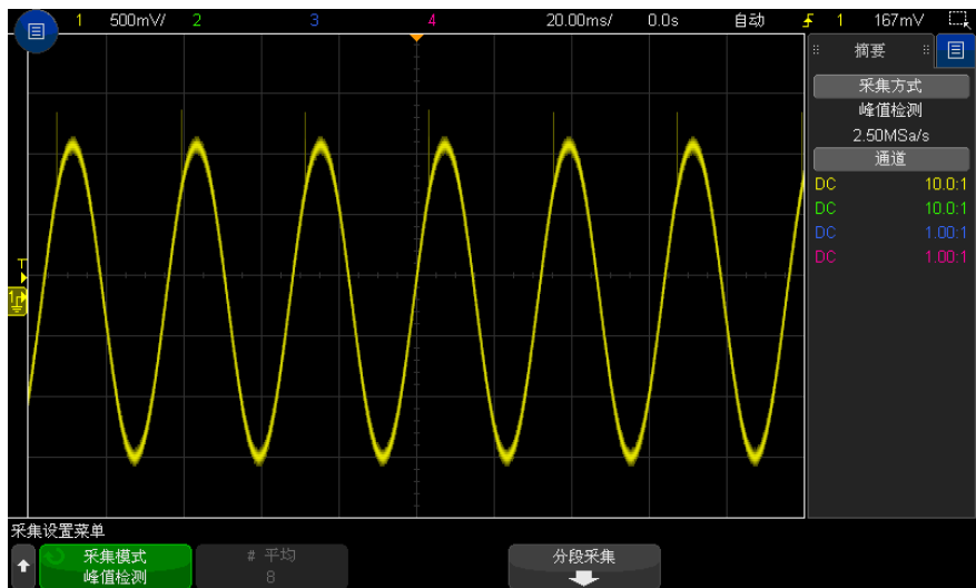
图 39 带毛刺的正弦波，峰值检测模式
