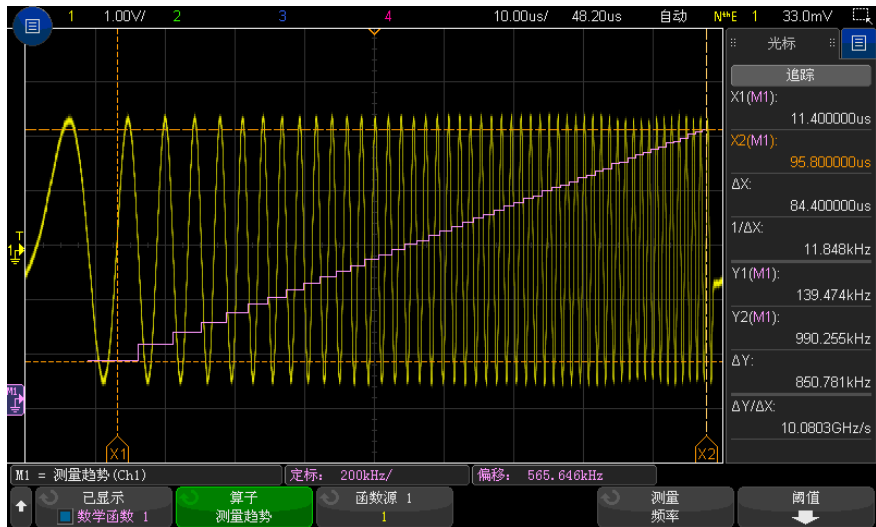
图 18 测量趋势示例
