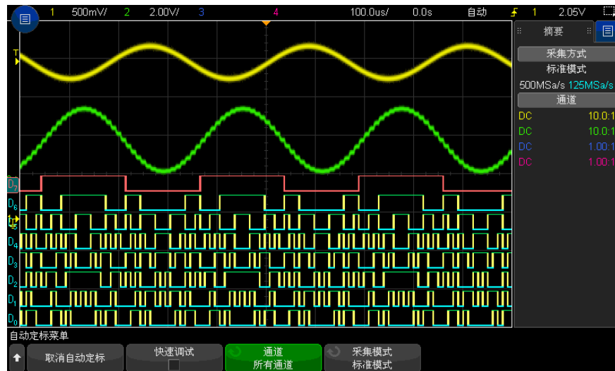
图 22 例如：数字通道的自动定标（仅限于 MS0 型号）
