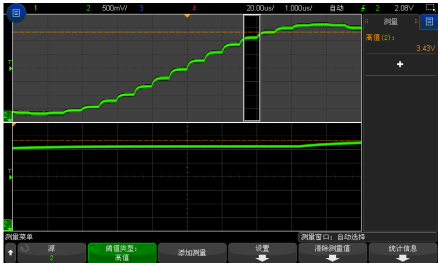
图 48 隔离高值测量区域
