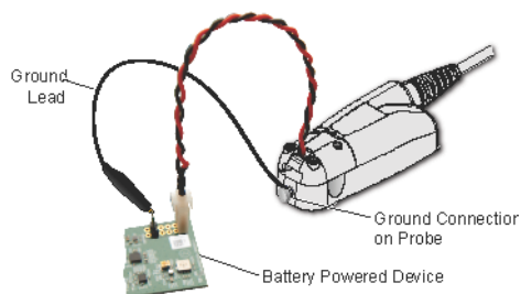
图 47 使用 N2820A 探头在电池供电的设备上进行测量
