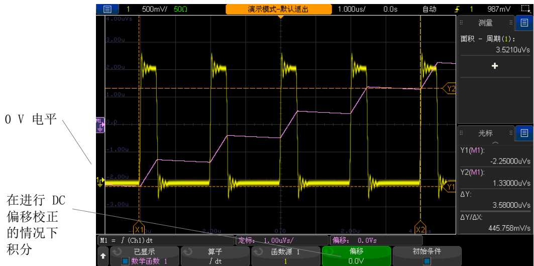
图 9 无信号偏移时的积分
