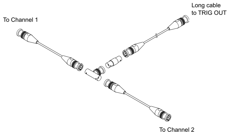
图 51 用于 2 通道示波器的用户校准电缆
