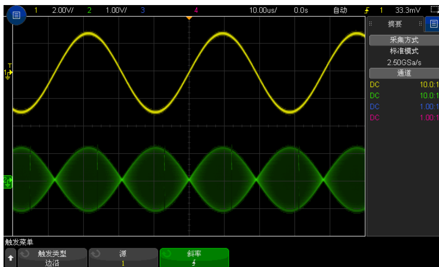
图 28 以 40% 亮度显示的调幅
