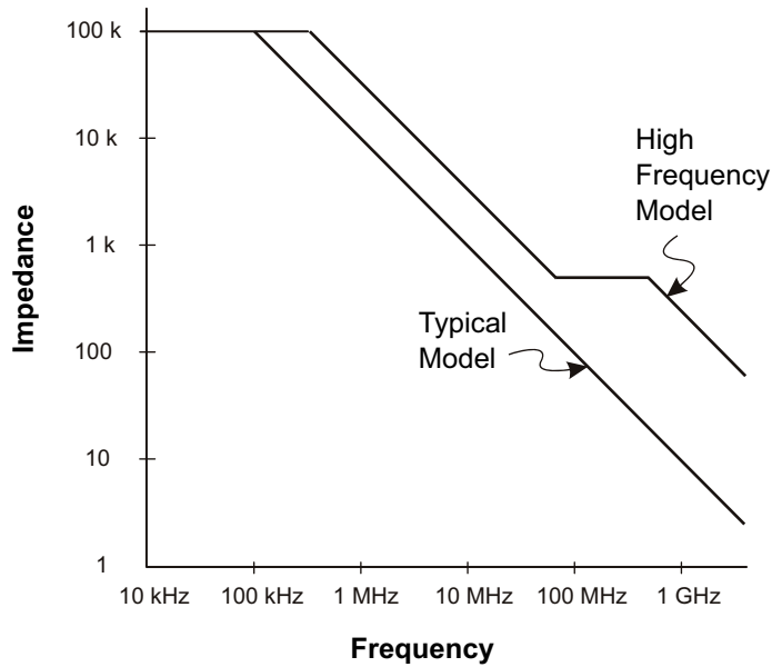
图 25 两个探头电路型号的阻抗和频率
