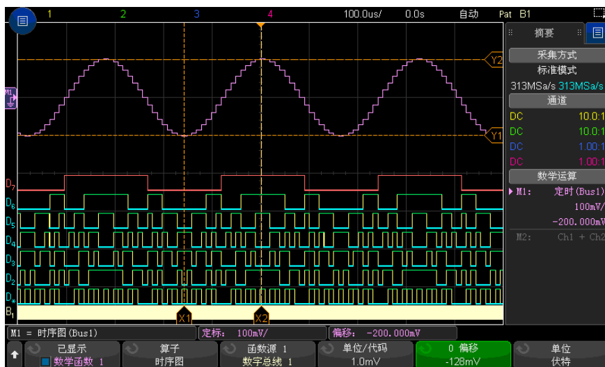
图 19 逻辑图总线时序示例
