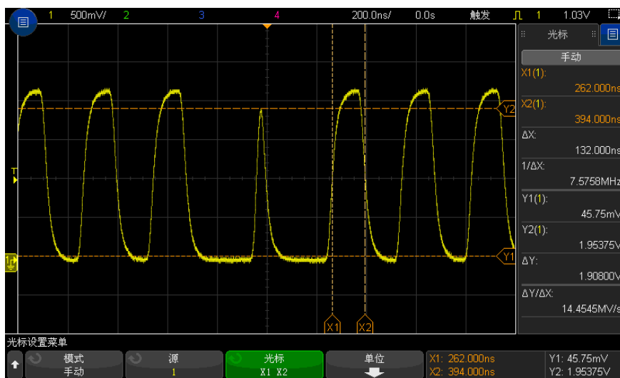
图 45 用光标测量脉冲宽度
