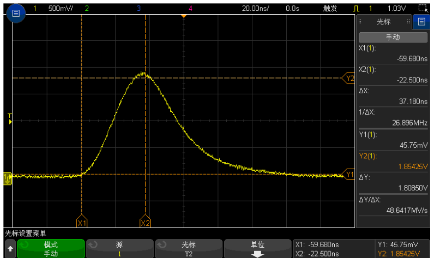
图 42 光标用于测量脉冲宽度而不是测量中阈点
