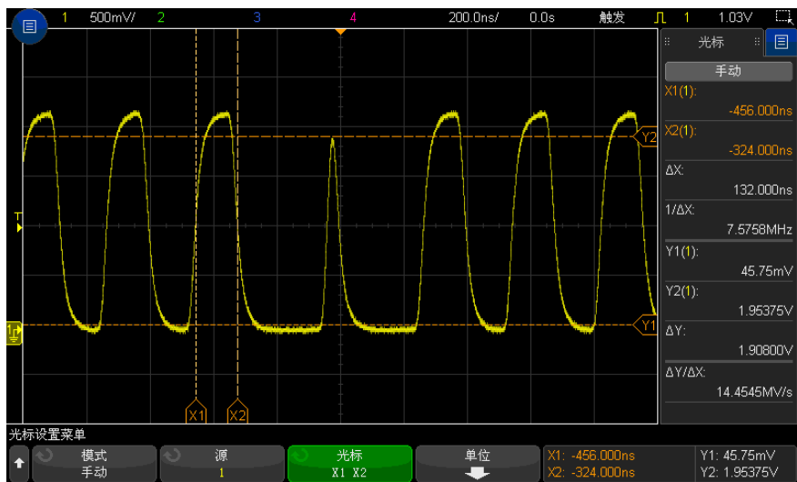
图 46 一起移动光标以检查脉冲宽度的变化
