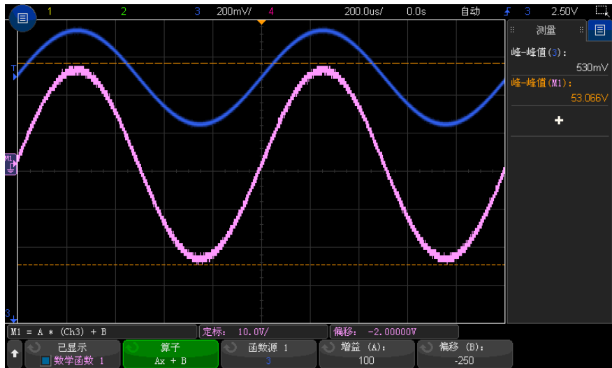
图 12 Ax + B 示例
