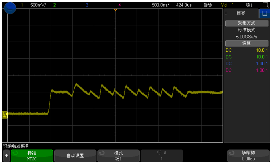
图 33 在彩色场 1 和彩色场 3 上交替触发
