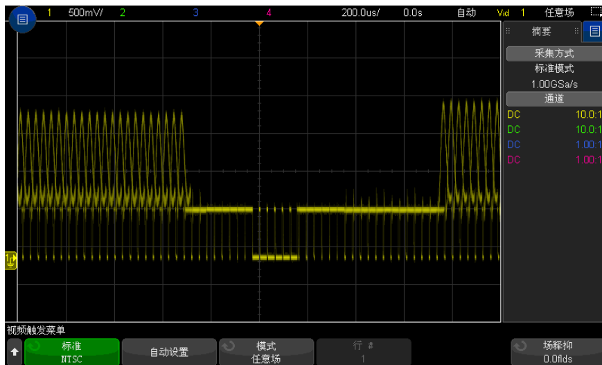
图 32 在所有场上触发
