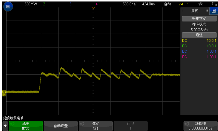
图 34 使用场释抑同步彩色场 1 或 3（场 1 模式）
