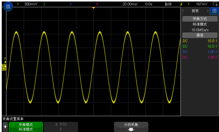
图 38 带毛刺的正弦波，正常模式
