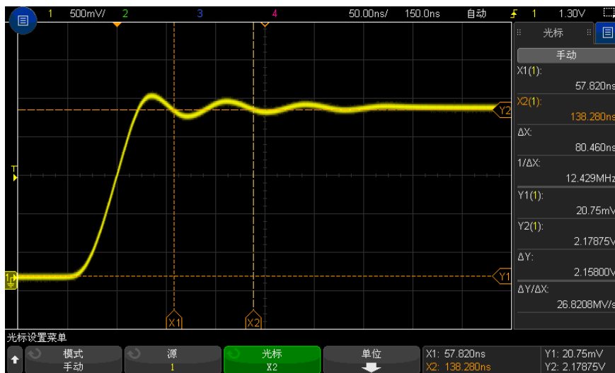
图 43 光标测量脉冲振铃频率
