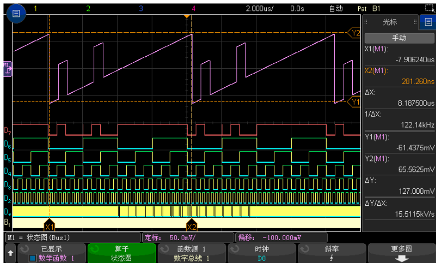
图 20 逻辑图总线状态示例
